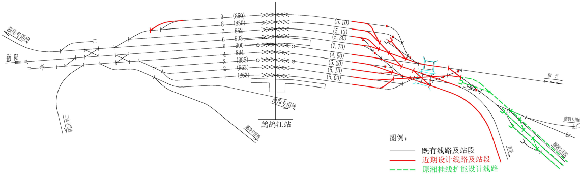
图 2.1-3 鹧鸪江站改扩建示意图
