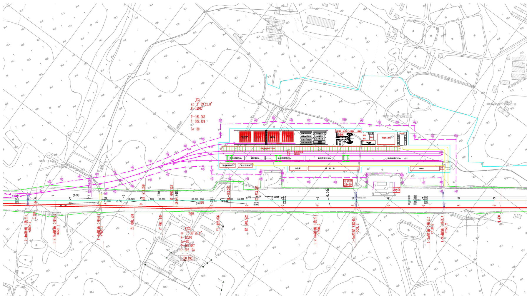
铺轨基地、制存梁场平面位置及外环境关系图
